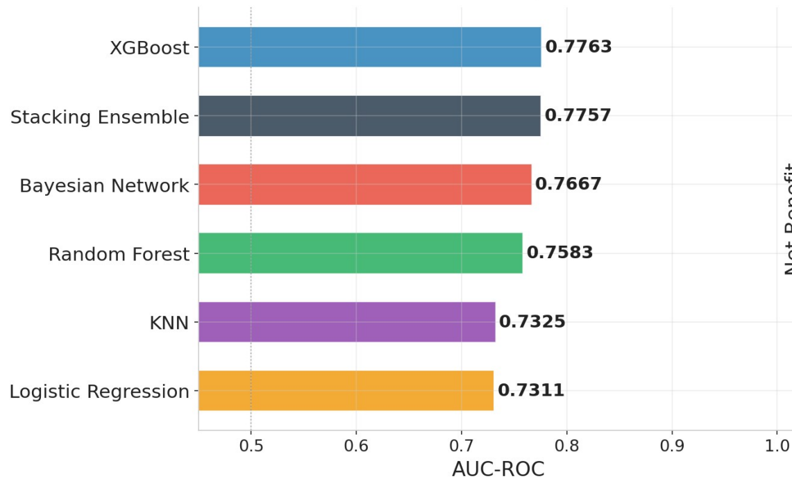
AUC-ROC Comparison
